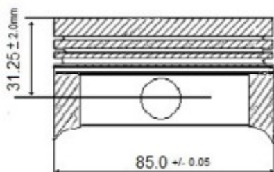
Dibujo pistón alternativo y medidas
