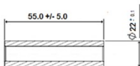
Dibujo perno pistón y medidas
