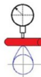
Rodillo medición árbol de levas 6.35 mm
