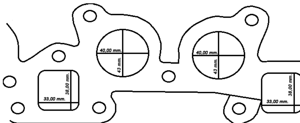
BASE DEL MULTIPLE FORD F 100, FASE 1 Y 2
