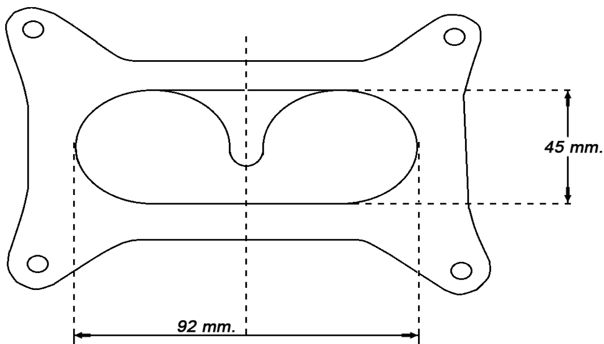
BASE DEL MULTIPLE FORD F 100, FASE 1 Y 2
